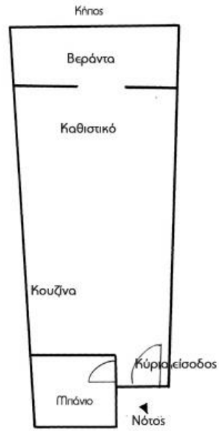
Κάτοψη
